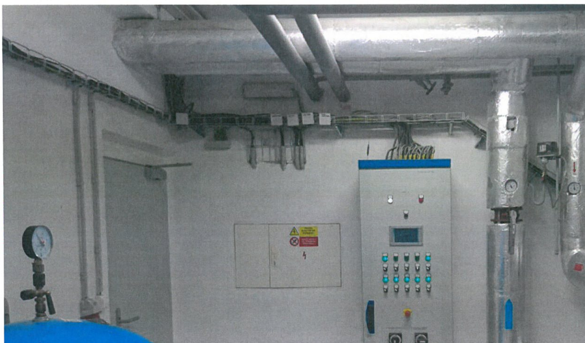
Pohled na úpravu vyvedených kabelů – stav po realizaci
